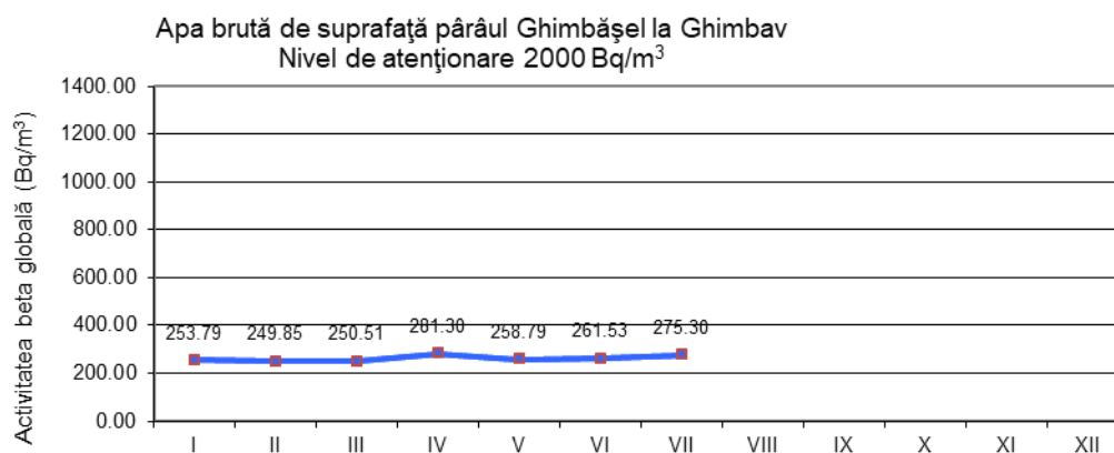
Figura 1.2.5: Activitatea beta globală imediată pentru apa de suprafață Pârâul Ghimbășel
