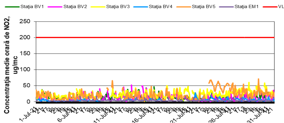
Figura 1.1.2.2.1. Evoluția mediilor orare de NO 2 în luna iulie
