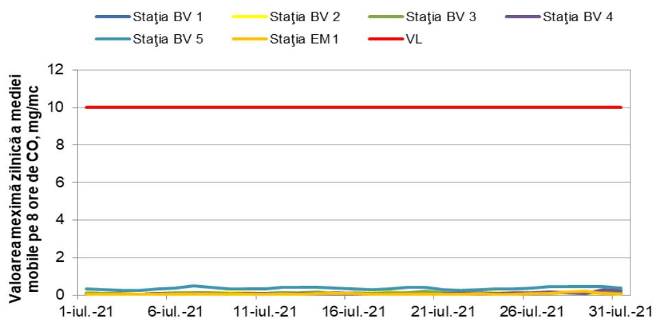
Figura 1.1.2.5.1. Evoluția maximelor zilnice ale mediei mobile de CO în luna iulie
