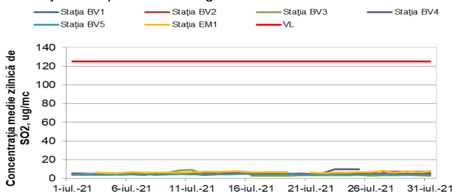
Figura 1.1.2.1.1. Evoluția mediilor zilnice de \text{SO}_2 în luna iulie
