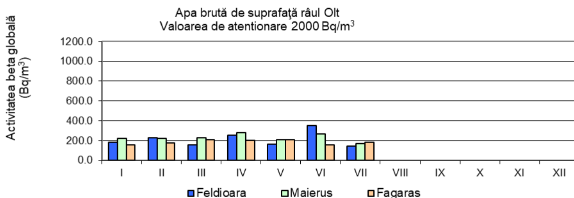
Figura 1.2.7: Activitatea beta globală la 5 zile pentru apa de suprafață Râul Olt
