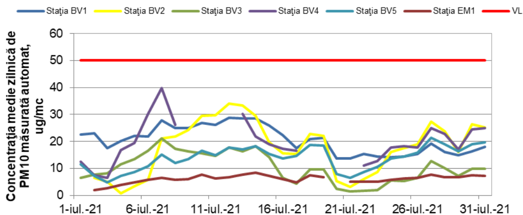
Figura 1.1.2.4.1. Evoluția mediilor zilnice de PM 10 în luna iulie
