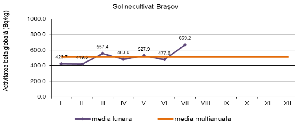
Figura 1.2.8: Activitatea beta globală la 5 zile pentru solul necultivat
