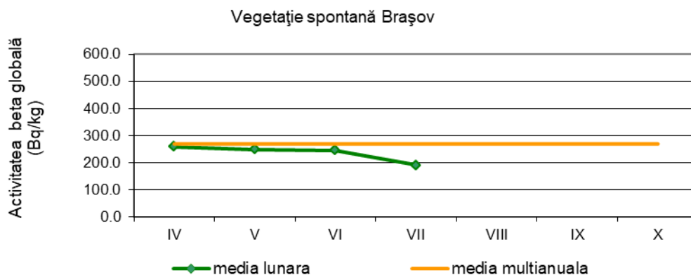
Figura 1.2.9: Activitatea beta globală la 5 zile pentru vegetația spontană
