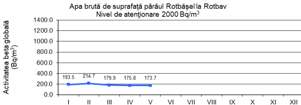
Figura 1.2.6: Activitatea beta globală la 5 zile pentru apa de suprafață-Pârâul Rotbășel
