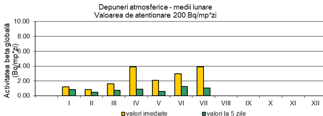
Figura 1.2.4: Activitatea beta globală pentru depuneri atmosferice
