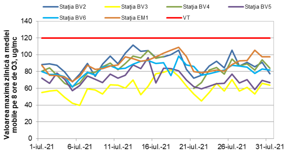
Figura 1.1.2.3.1. Evoluția maximelor zilnice ale mediilor mobile pe 8 ore de \text{O}_3 în luna iulie
