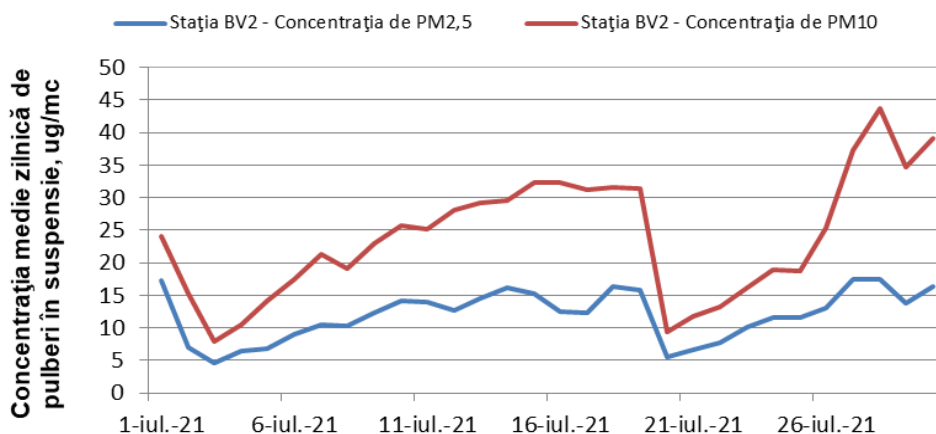
Figura 1.1.2.4.4 Evoluția mediilor zilnice de PM 2,5 și PM10 în luna iulie
