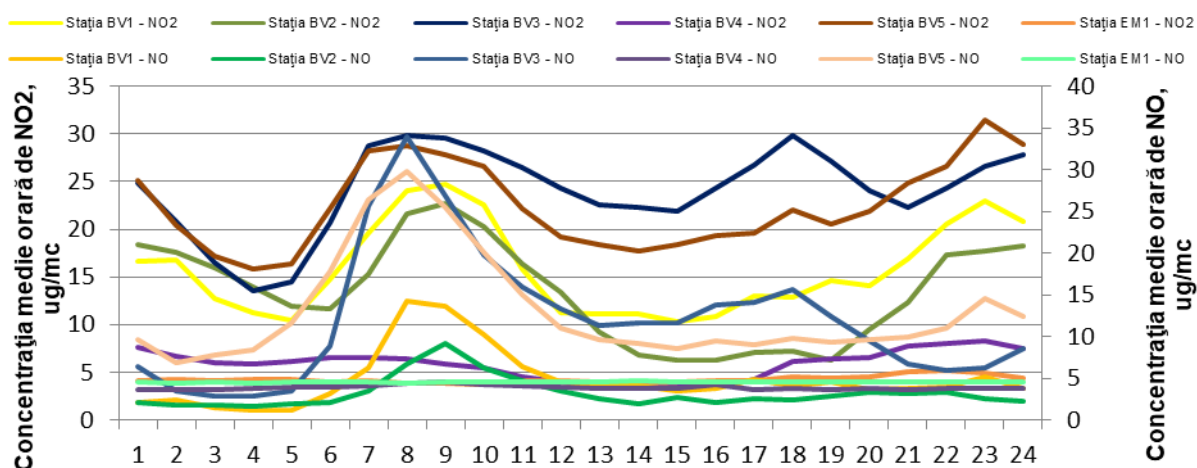
Figura 1.1.2.2.2. Ciclul zilnic al NO 2 și NO
