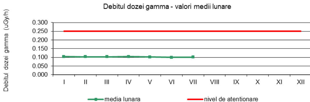
Figura 1.2.3: Debitul dozei gamma în aer
